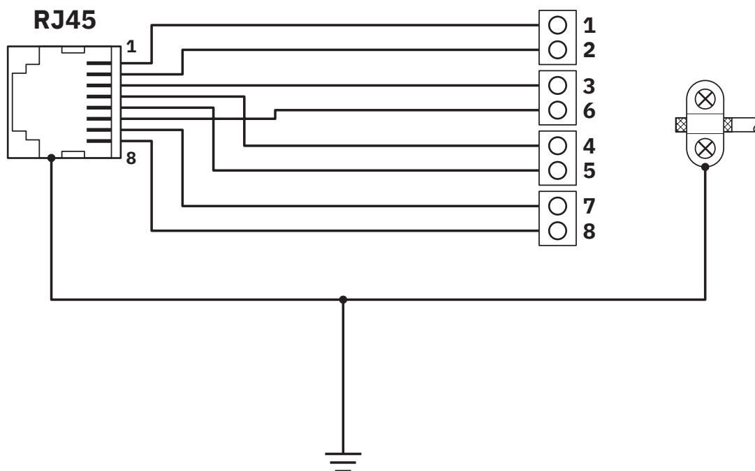
schakelschema
