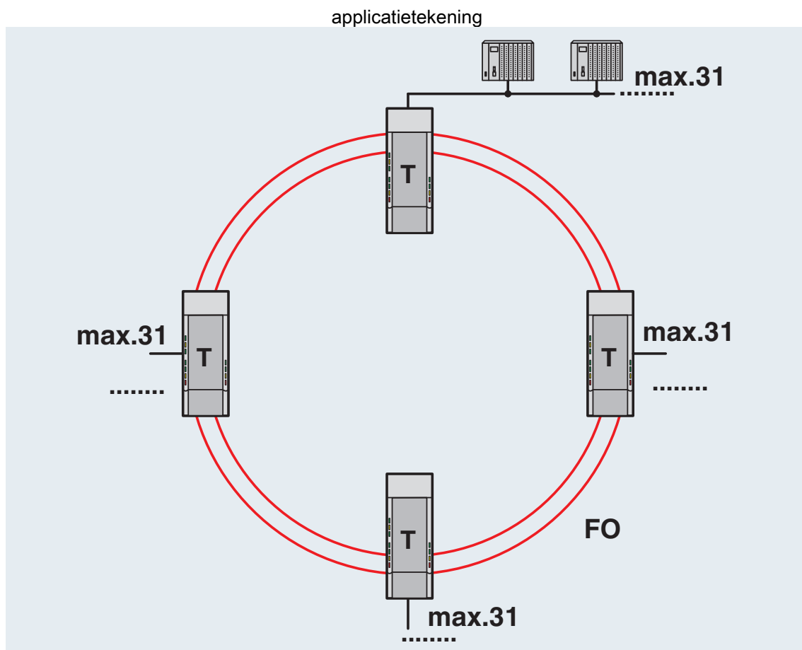
Redundante glasvezelring
