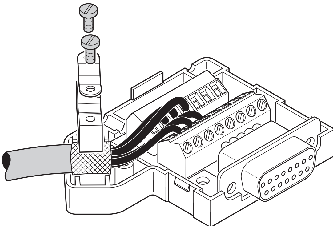
Aansluiting van de kabels
