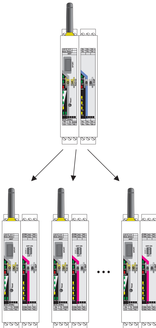
functietekening
