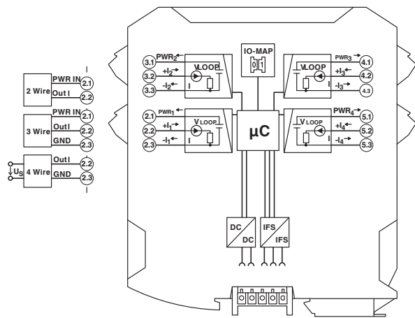
schakelschema
