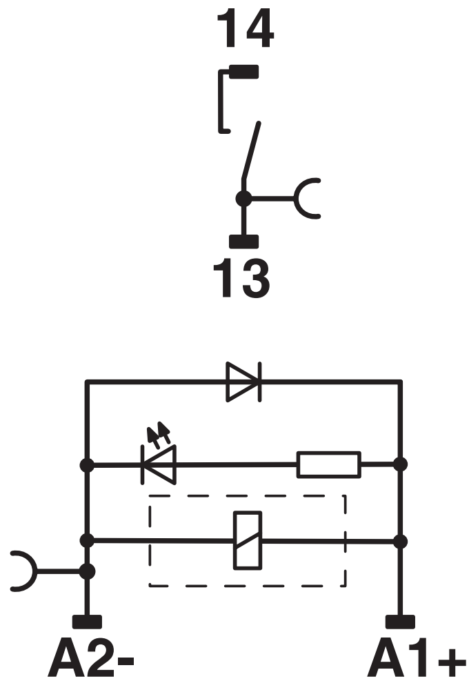
schakelschema
