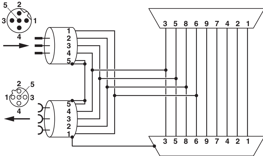
Functieschakelschema SUBCON-PLUS-PROFIB/...M12
