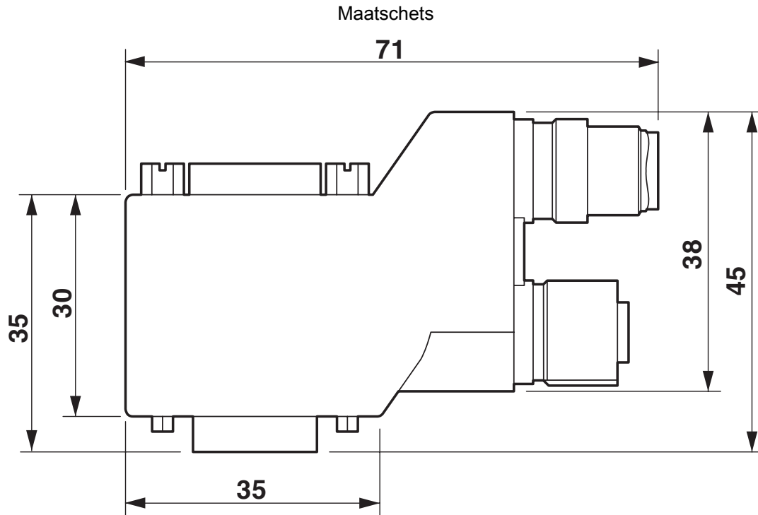
Maatschets SUBCON-PLUS...90...M12, korte 90°-variant
