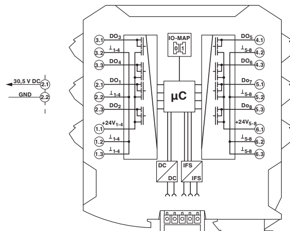
schakelschema
