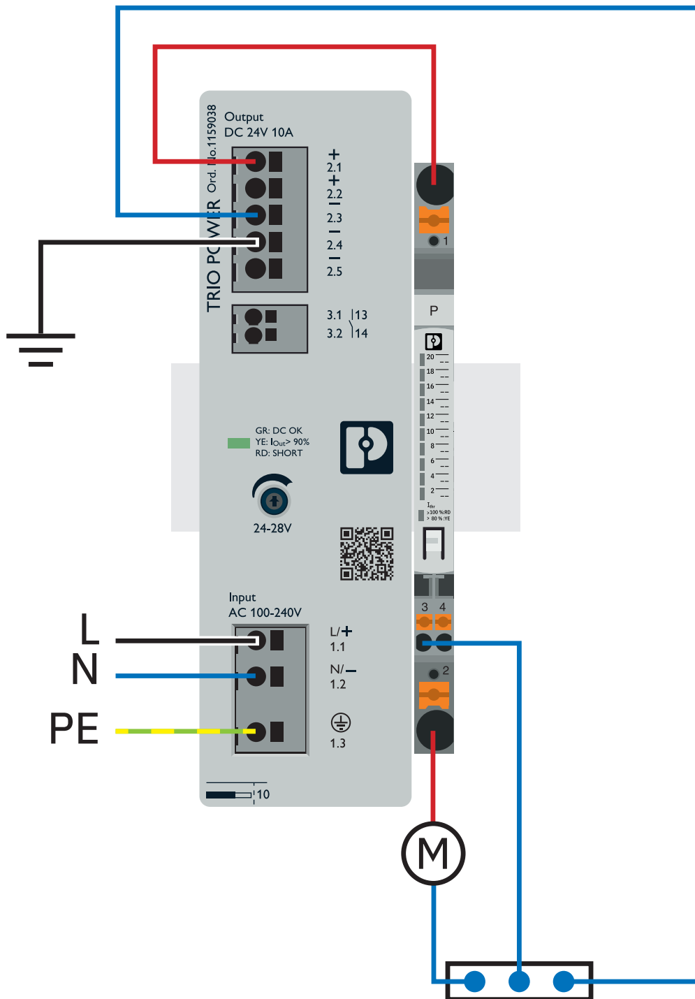
applicatietekening
