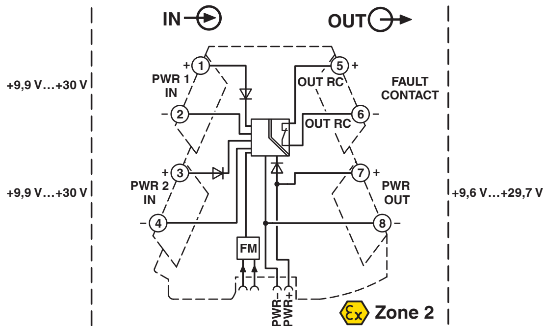
blokschema
