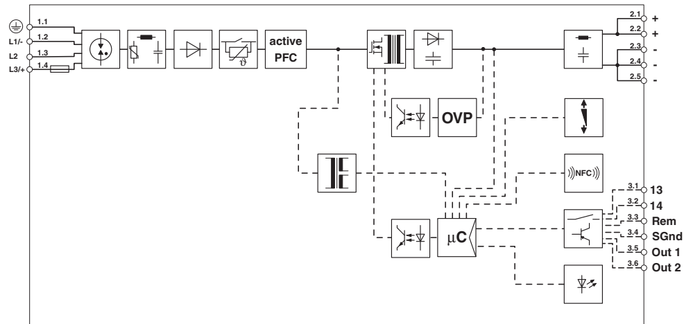
blokschema
