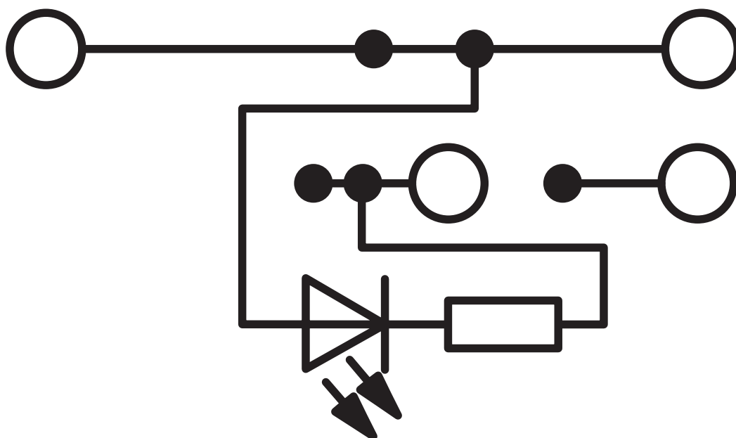
schakelschema
