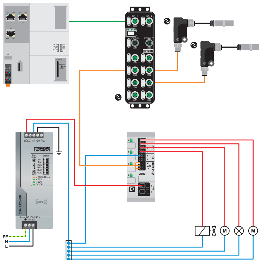
applicatietekening
