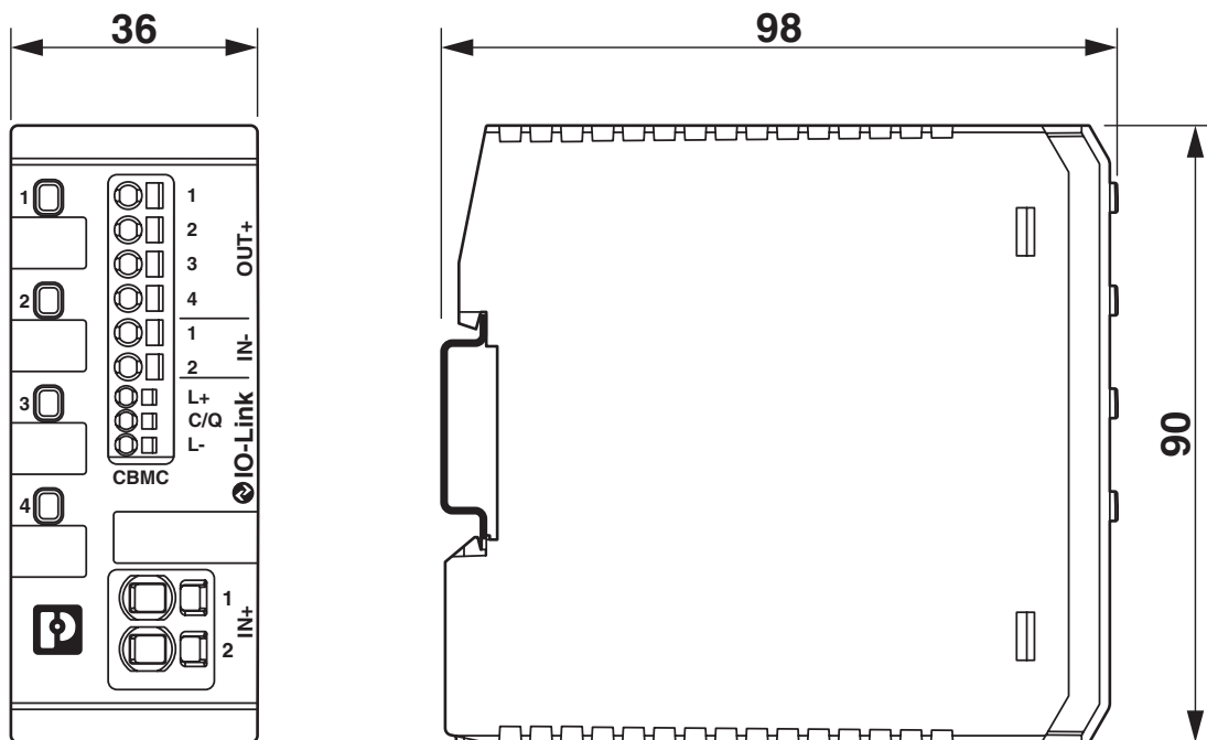
Maatschets
