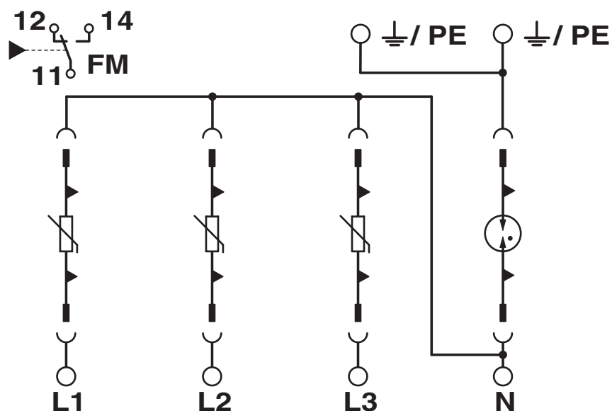
schakelschema
