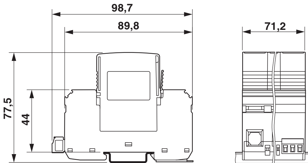
Maatschets
