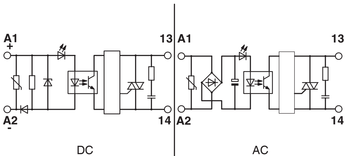
schakelschema
