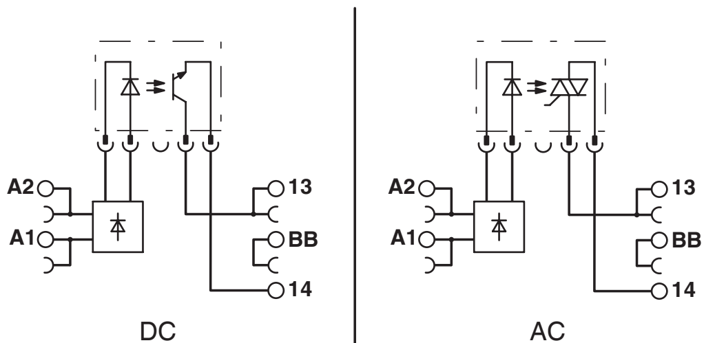
schakelschema
