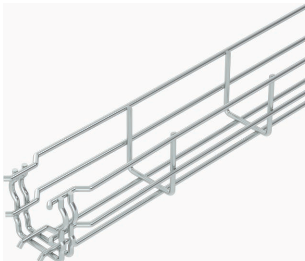
Draadgoot met aangevormde verbinder zijhoogte 55 mm.
