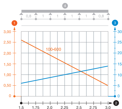
Belastingsdiagram kabelgoot type SKSU 60
