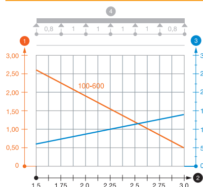
Belastingsdiagram kabelgoot type SKSMU 60
