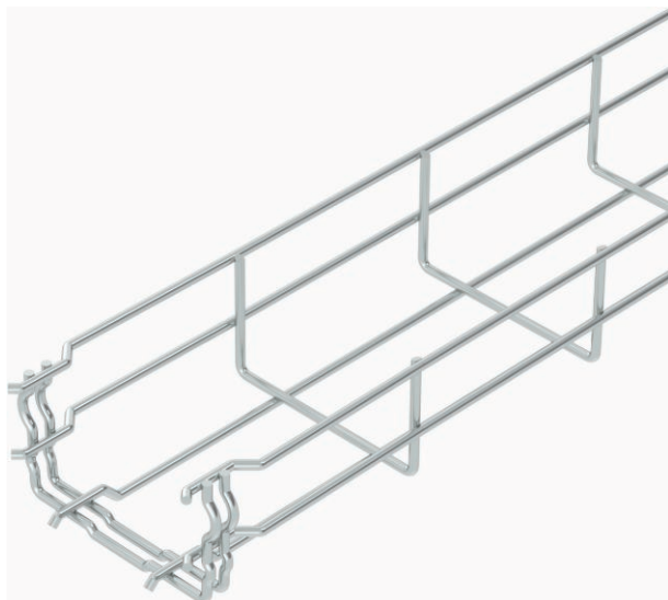
Draadgoot met aangevormde verbinder zijhoogte 55 mm.
