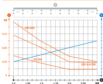
Belastingdiagram draadgoot GR-Magic type GRM 55
