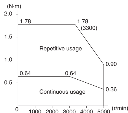
R88M-G20030L
